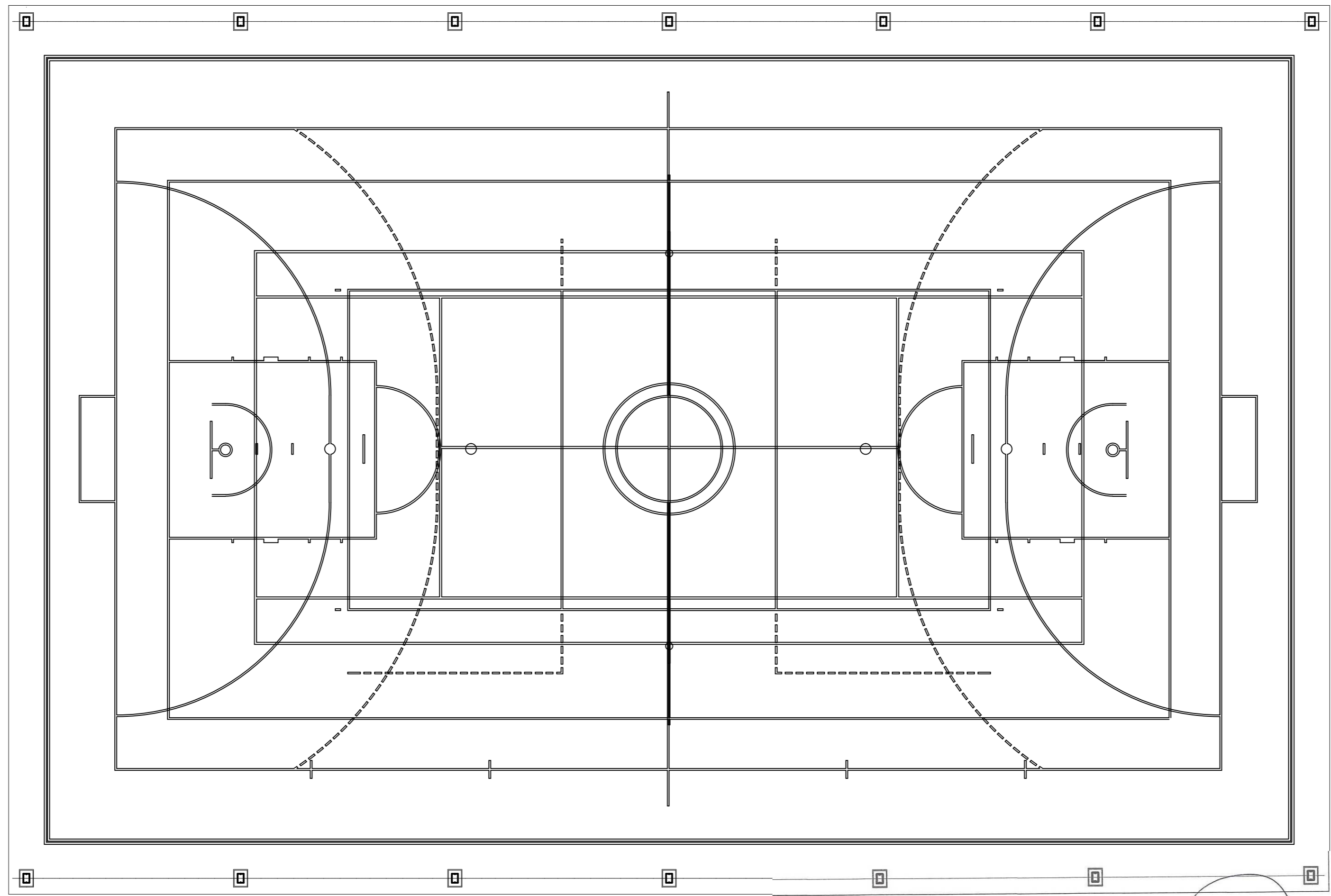
DEMARCAÇÃO POLIESPORTIVA 1:75
